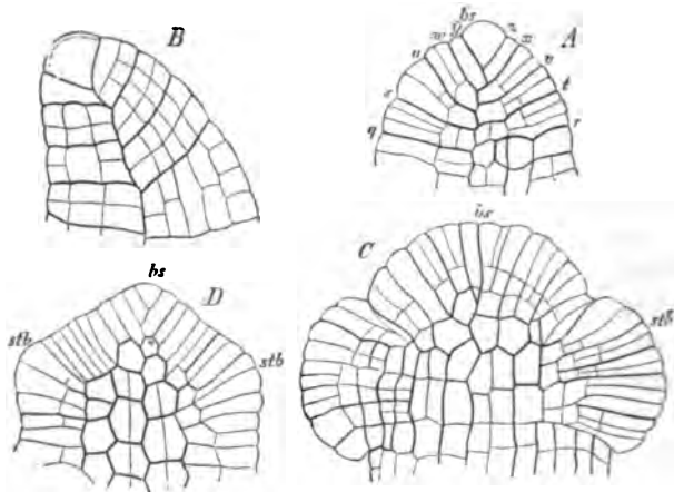
Fig. 134. — Développement de la feuille du Marsilia Drummondii d'après M. Hanstein. A, C, D, vu par la face interne; B section longitudinale perpendiculaire de A; bs, sommet de la feuille; q-s, les segments de la cellule terminale; stb, les lobes latéraux du limbe, dans leur premier âge.
